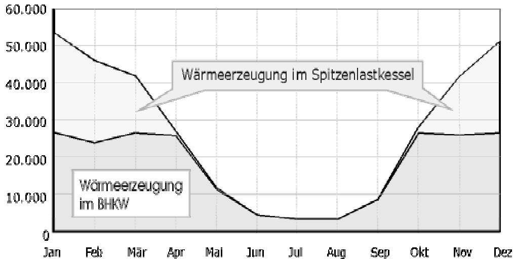
Wärmebedarf und Wärmeerzeugung im Hotel Bären (Wärmeerzeugung in kWh/Monat)
